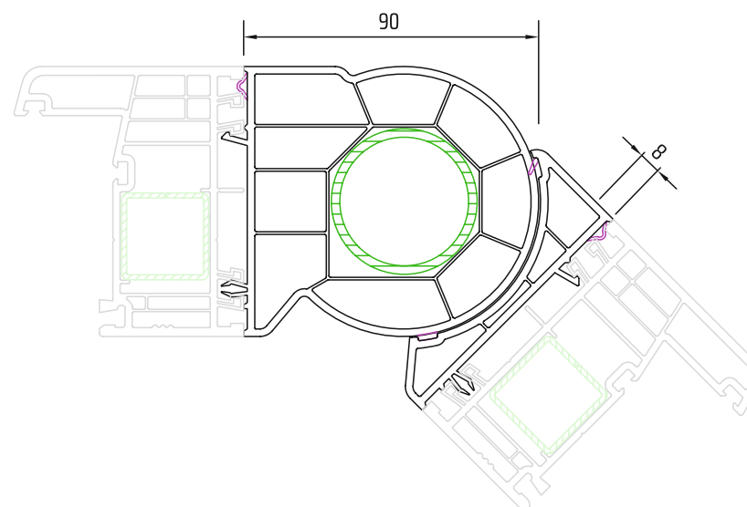
łącznik 5206
