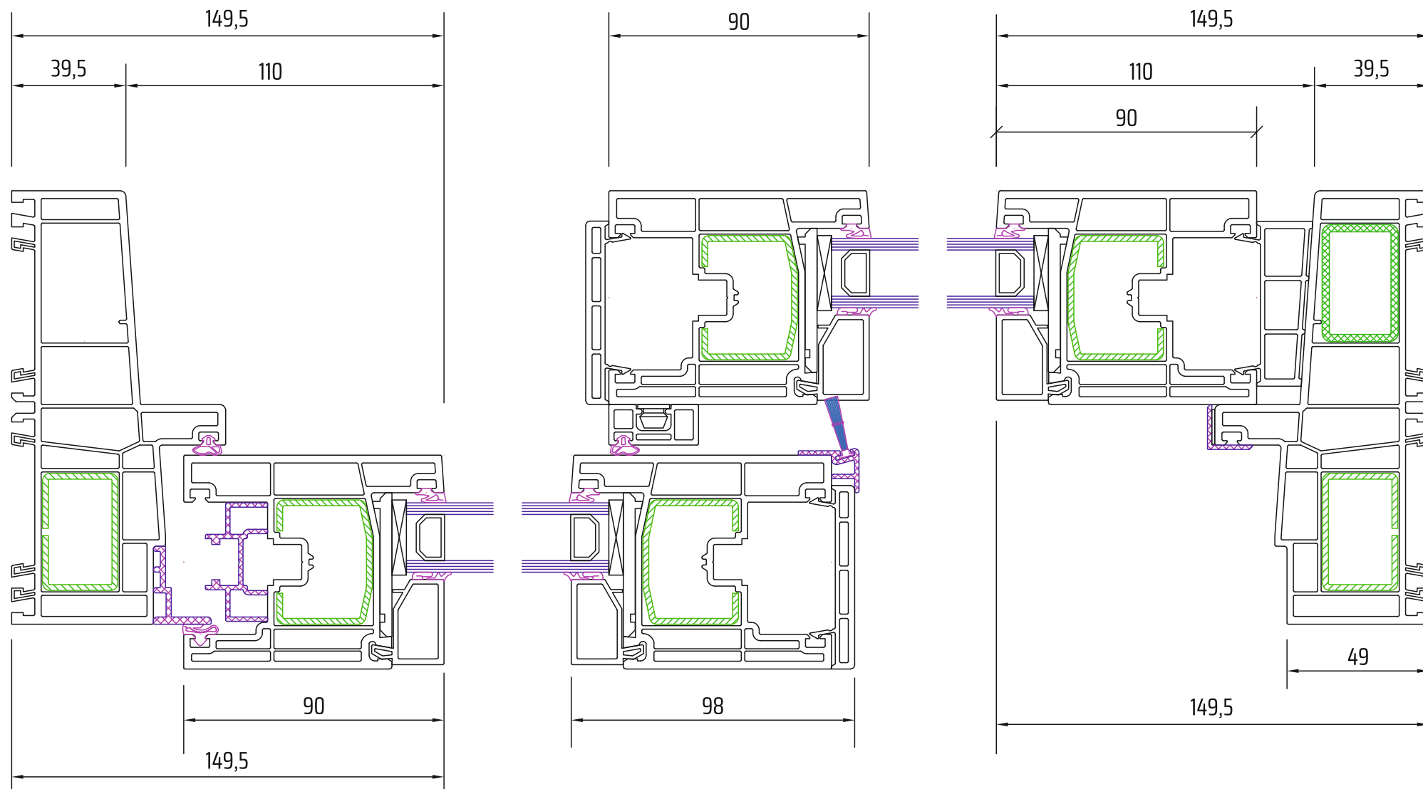
Przekrój poziomy
