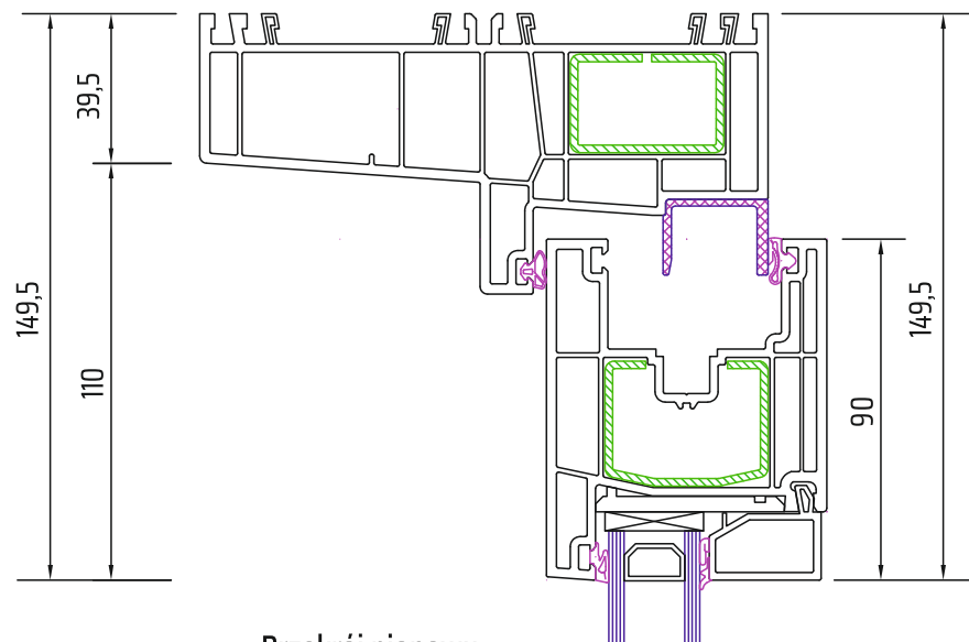
Przekrój pionowy części ruchomej
