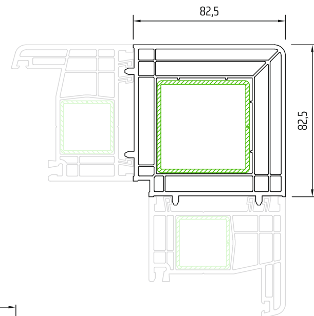
łącznik 2304
