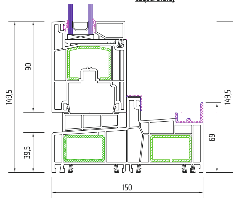
Przekrój pionowy części stałej
