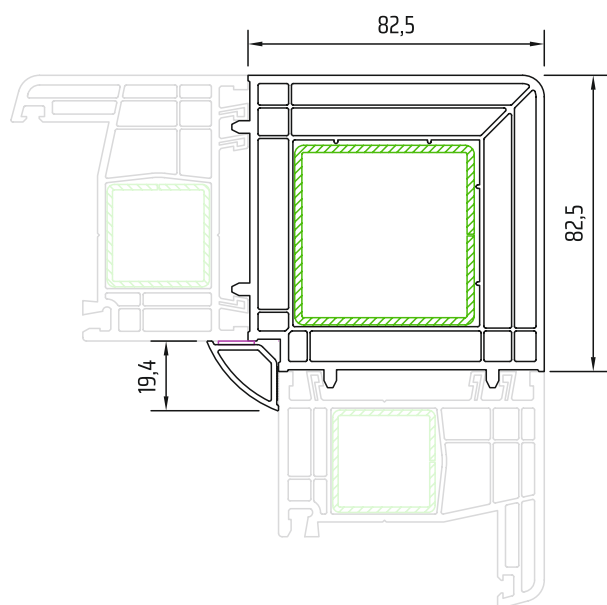
łącznik 2304+2325
