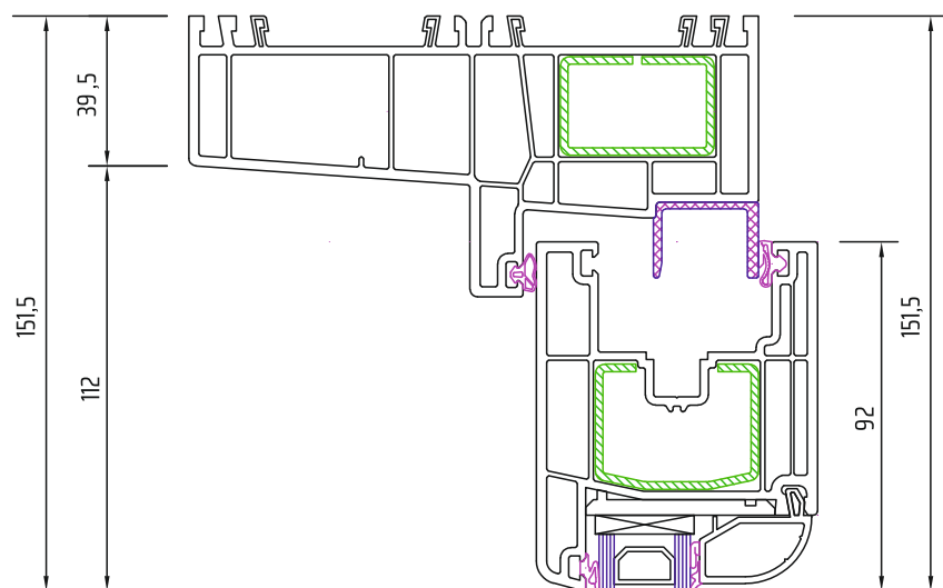
Przekrój pionowy części ruchomej
