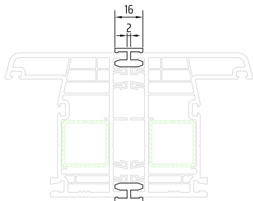
łącznik piórowy
