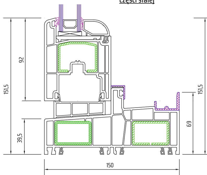
Przekrój pionowy części stałej
