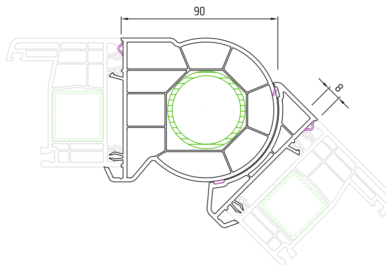
łącznik 2233/2234
