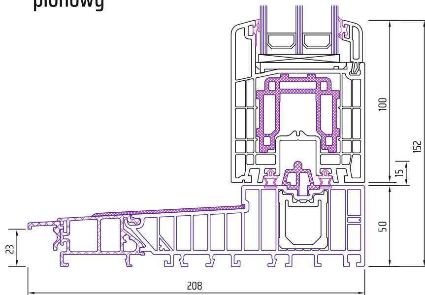
Przekrój pionowy
