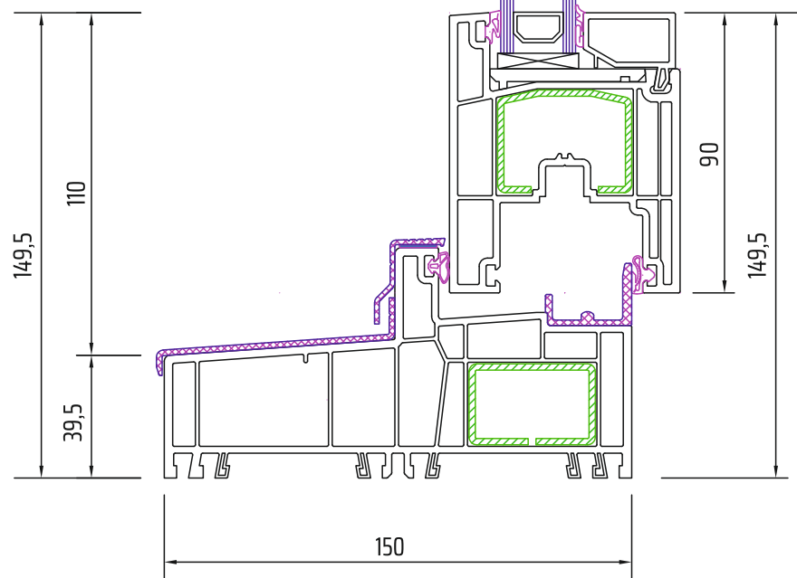
Przekrój pionowy części ruchomej
