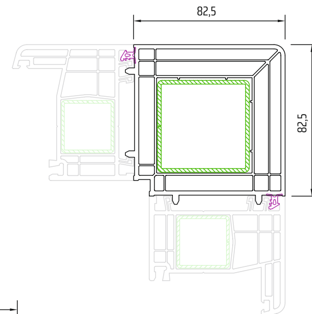
łącznik
